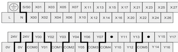
H3U-1616MR/T-XA 机型端子图
