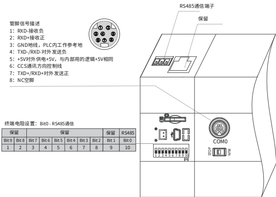
H3U-1010MR/T-XA、H3U-1616MR/T-XA、H3U-2416MR/T-XA 相关通信配置示意图
