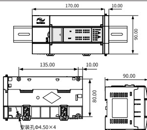
图 4 H3U-1010MR/T-XA、H3U-1616MR/T-XA、H3U-2416MR/T-XA 产品尺寸 (单位: mm)
