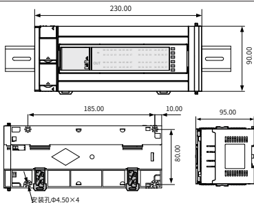
图 3 H3U-3232MR/T-XA、R/H3U-3624MR/T-XA 产品尺寸 (单位: mm)
