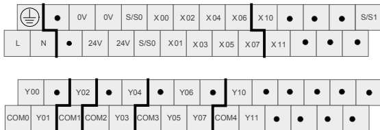
H3U-1010MR/T-XA 机型端子图
