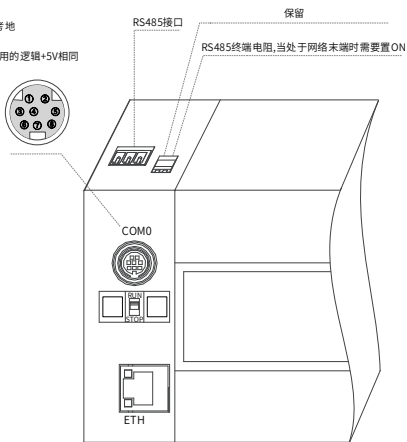
H3U-3232MR/T-XA、H3U-3624MR/T-XA 相关通信配置示意图
